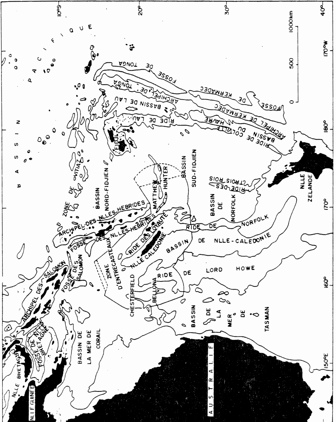
Fig. 1 - Carte bathymétrique du Sud-Ouest Pacifique
